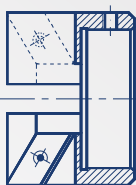
Pipe cutter 30° ID 25 - OD 58 mm Item 091501102
