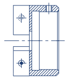
Pipe cutter 0° ID 11 - OD 22 mm Item 091505347
