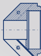
Pipe cutter 0° ID 25 - OD 66 mm Item 010007079
